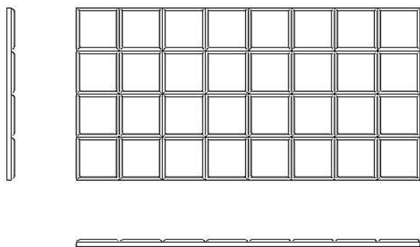
Панель “Линия” ГВ 145x145мм Ш1.0 Ф5/4 Размеры 1160x580x20/25мм
