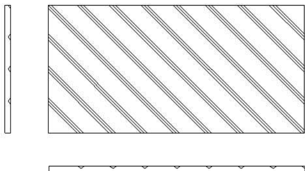
Панель “Линия” Д 145мм Ш1.0 БФ Размеры 1160x580x20/25мм
