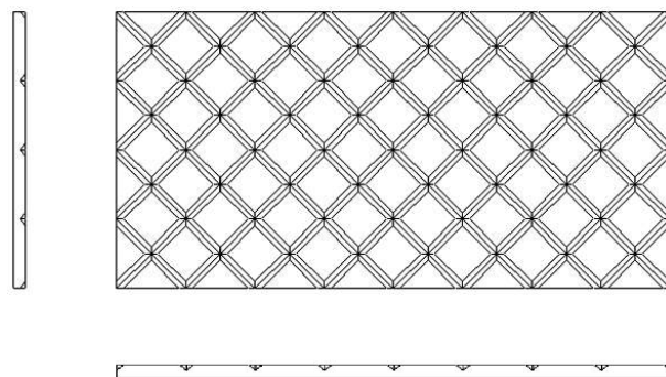
Панель “Линия” ДГВ 145x145мм Ш1.0 БФ Размеры 1160x580x20/25мм
