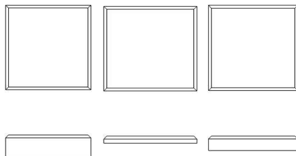
Панель “Кнопка” 15/20/25/50/75мм Ш1.0 Ф5 Размеры 580x580мм; 290x290мм
