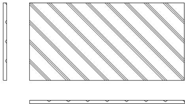
Панель “Шедр 3D” Д 145мм 450W/25 Ш1.0 Ф0/4 Размеры 1160x580x25мм
