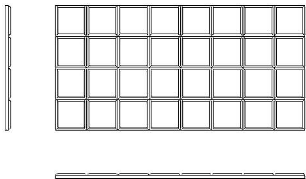
Панель “Шедр 3D” ГВ 145x145мм 450W/25 Ш1.0 Ф10/4 Размеры 1160x580x25мм
