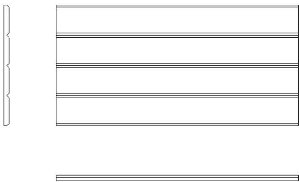
Панель “Шедр 3D” Г 145мм 450W/25 Ш1.0 Ф10/2 Размеры 1160x580x25мм
