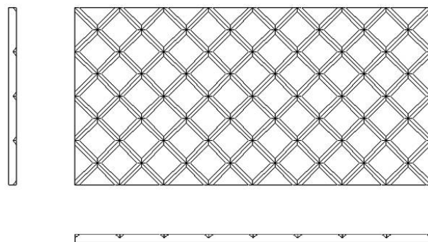
Панель “Шедр 3D” ДГВ 145x145мм 450W/25 Ш1.0 Ф0/4 Размеры 1160x580x25мм
