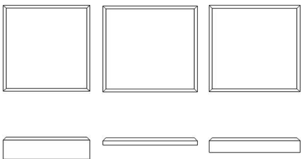
Панель “Шедр 3D” 25/50/75мм 450W Ш1.0 Ф10/4 Размеры 580x580x25/50/75мм; 290x290x25/50/75мм
