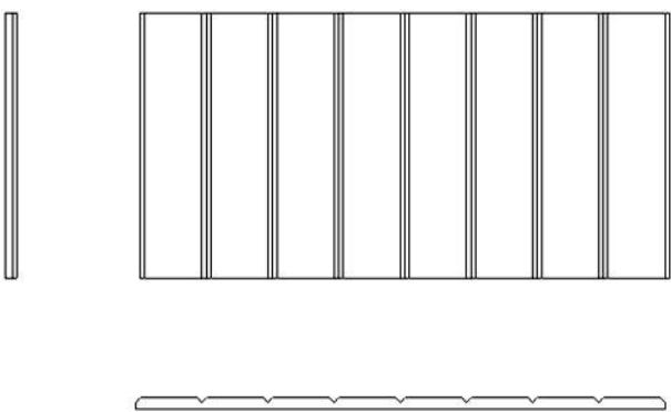
Панель “Шедр 3D” В 145мм 450W/25 Ш1.0 Ф10/2 Размеры 1160x580x25мм
