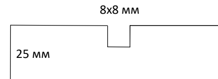
Сечение фрезеровки для панели толщиной 25мм
